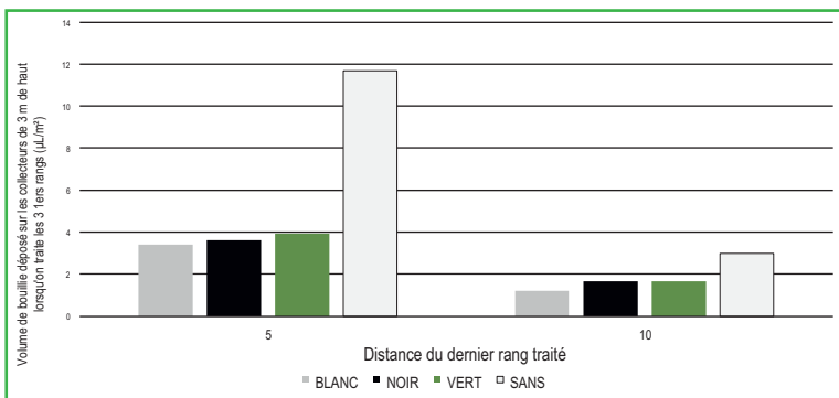
Evaluation de l'effet antidérive des différents filets
